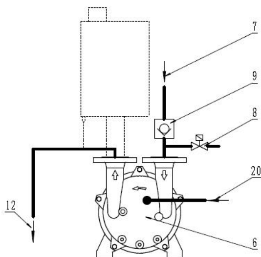
Рисунок 1. Проточный метод (слева); сепаратор и частичная рециркуляция
