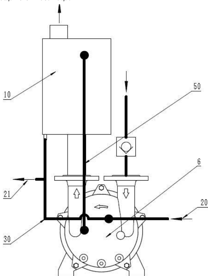
Рисунок 2. 6) вакуумный насос; 10) сепаратор; 20) подача рабочей жидкости; 21) слив рабочей жидкости; 30) линия циркуляции рабочей жидкости; 50) линия защиты от кавитации.
