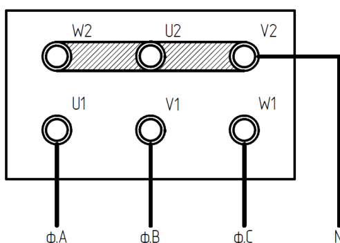
Подключение по схеме «звезда»
