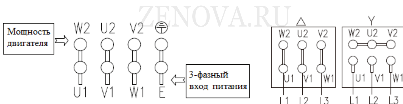
Рис. 4 – Схема подключения 3 проводов (слева) и 6 проводов (справа) трехфазного электродвигателя насосов серии VRD
