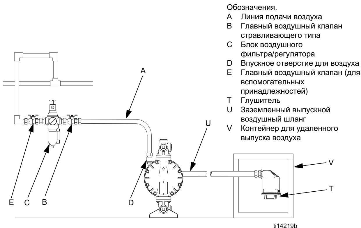
Рис. 3. Вытяжная вентиляция
